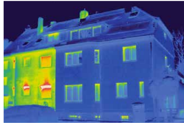
Deutlich zu erkennen: Eine gedämmte und ungedämmte Außenwand an einem Mehrfamilienhaus.
